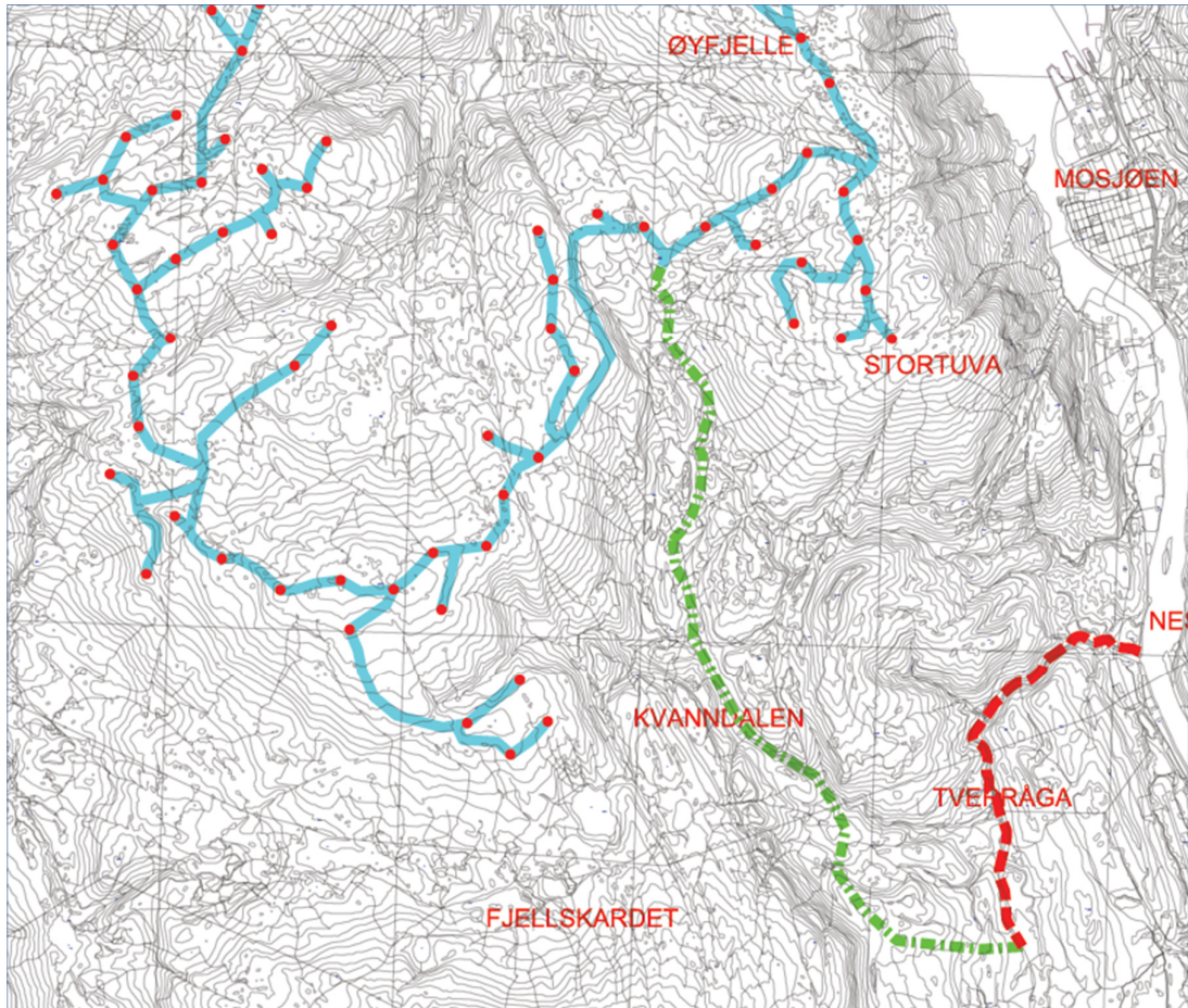
Figur 3-7: Vegtilknytning Øyfjellet vindkraftverk, søndre del.
