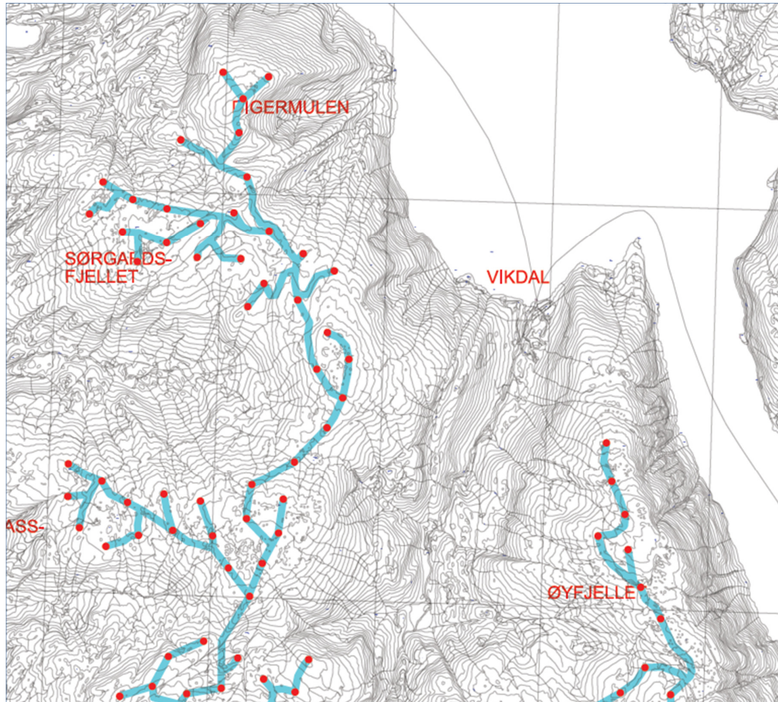
Figur 3-8: Vegtilknytning Øyfjellet vindkraftverk, nordre del.
